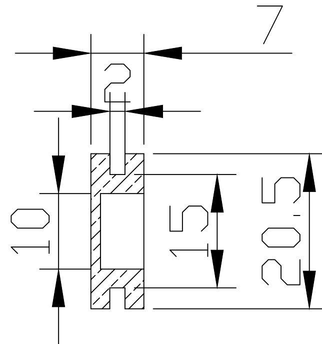
Sezione A-A
