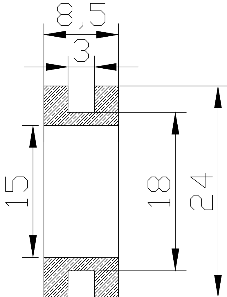
Sezione A-A
