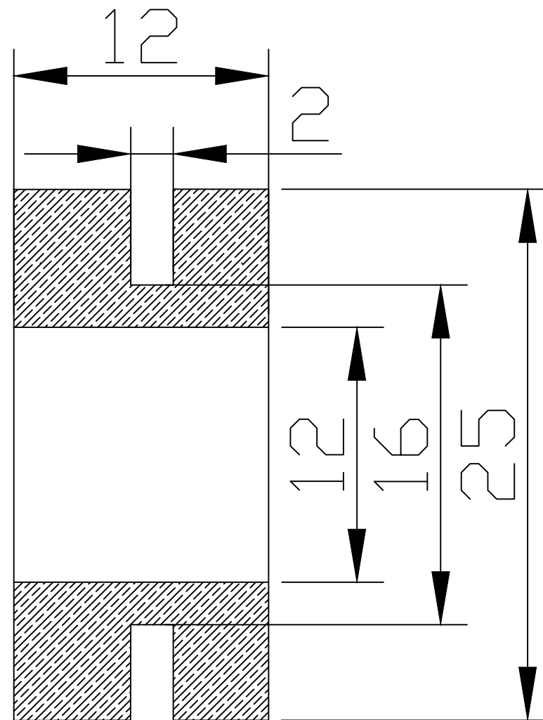
Sezione A-A
