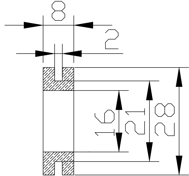
Sezione A-A
