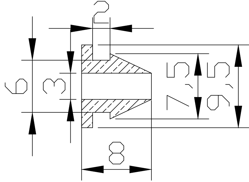
Sezione A-A
