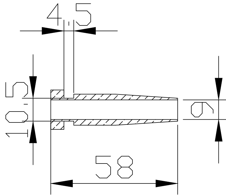
Sezione A-A
