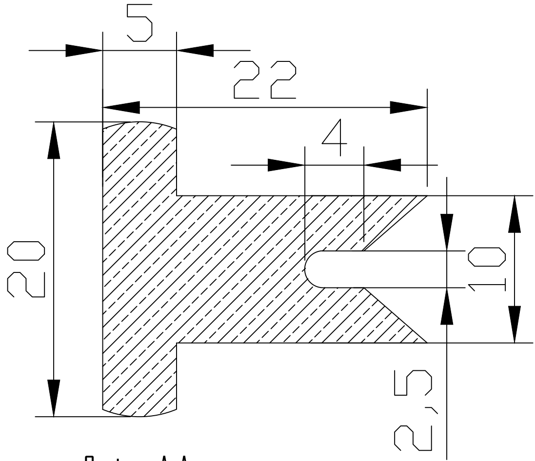
Sezione A-A
