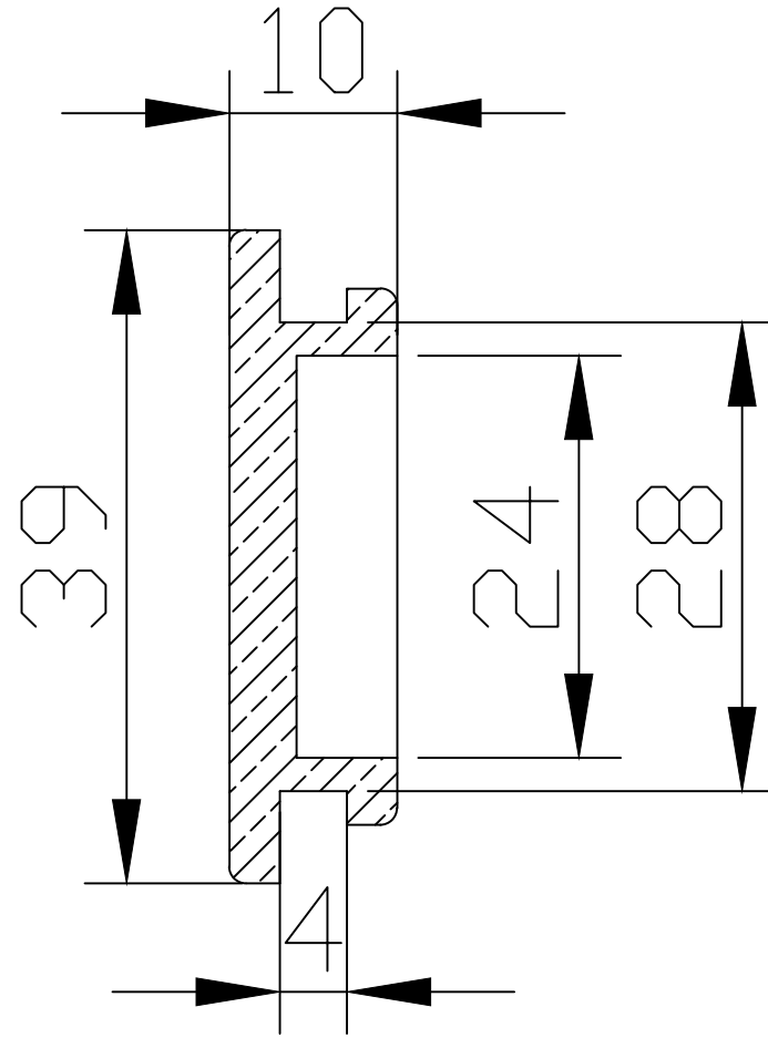
Sezione A-A
