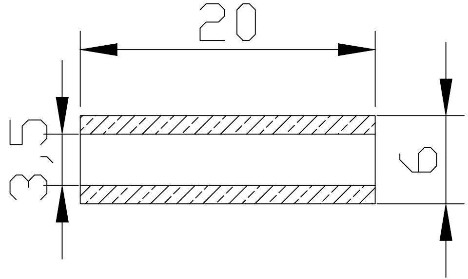
Sezione A-A
