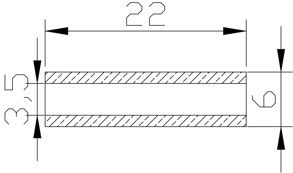
Sezione A-A
