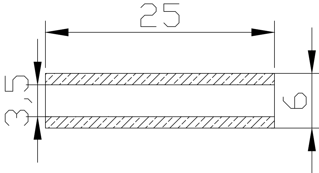
Sezione A-A
