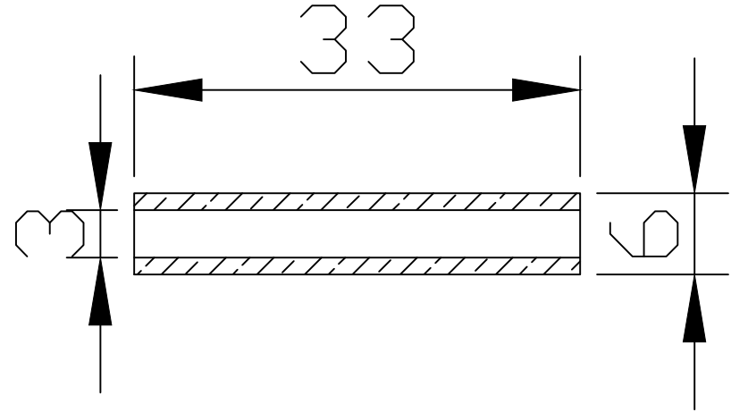
Sezione A-A
