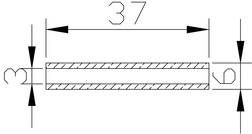
Sezione A-A
