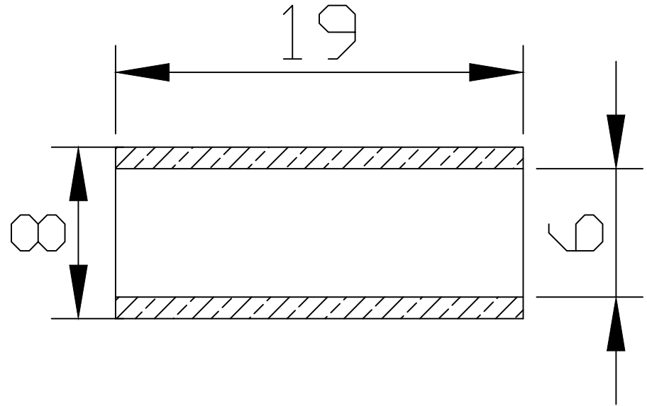
Sezione A-A
